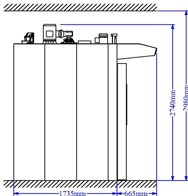
VISTA LATERAL
